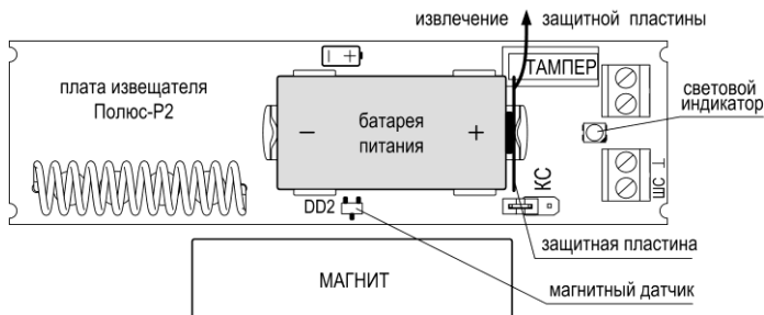
Рис.10 Плата извещателя Полюс-Р2
