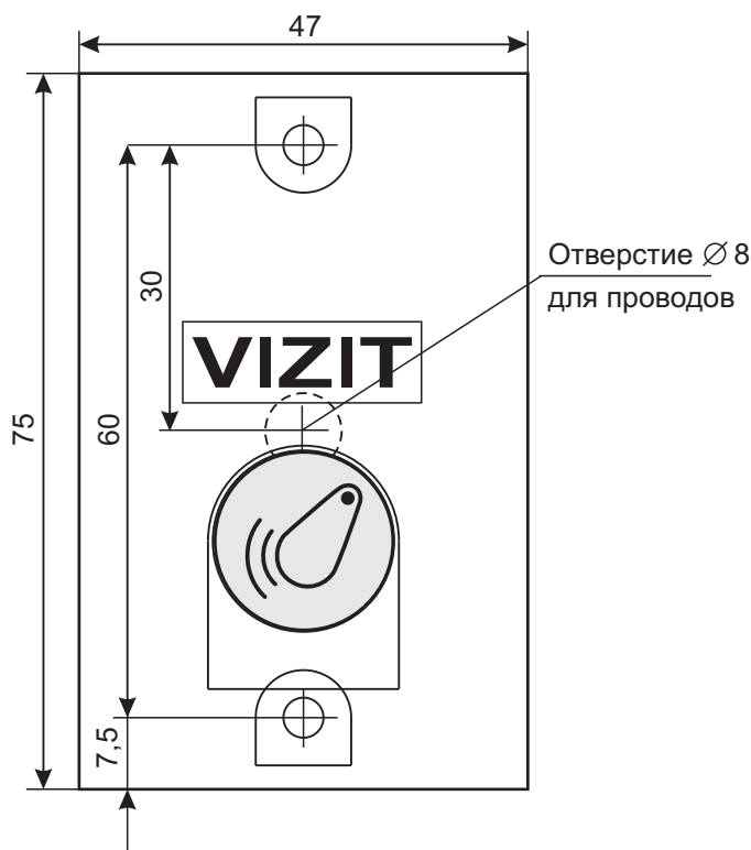
Рисунок 1 - Установочные размеры считывателя RD-3
